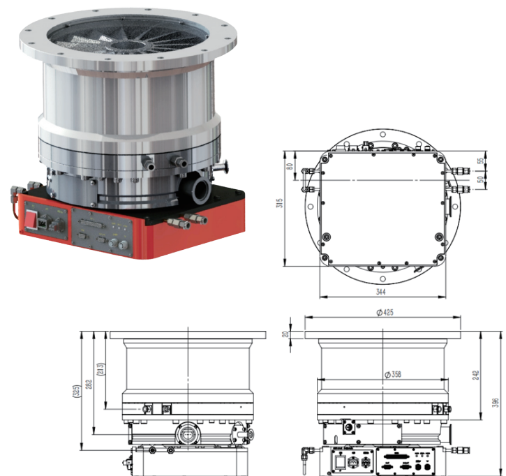
外形图
