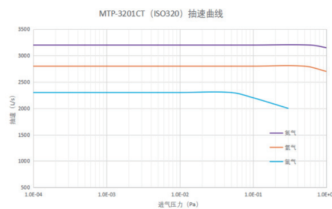
抽速及流量曲线
