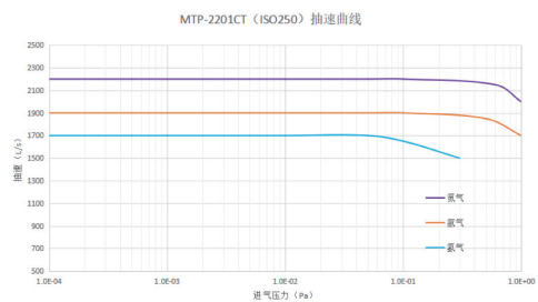
抽速及流量曲线
