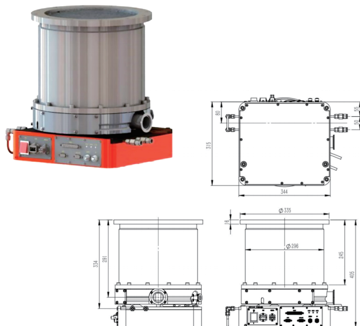
外形图
